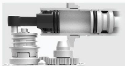
Bielva de manivela para máxima estabilidad.
